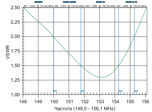
График КСВ А-1000MV
