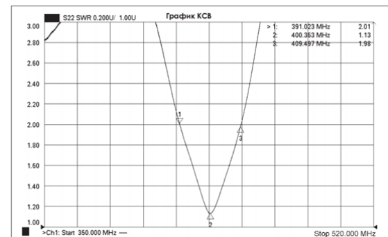
График КСВ А-200МУ-N
